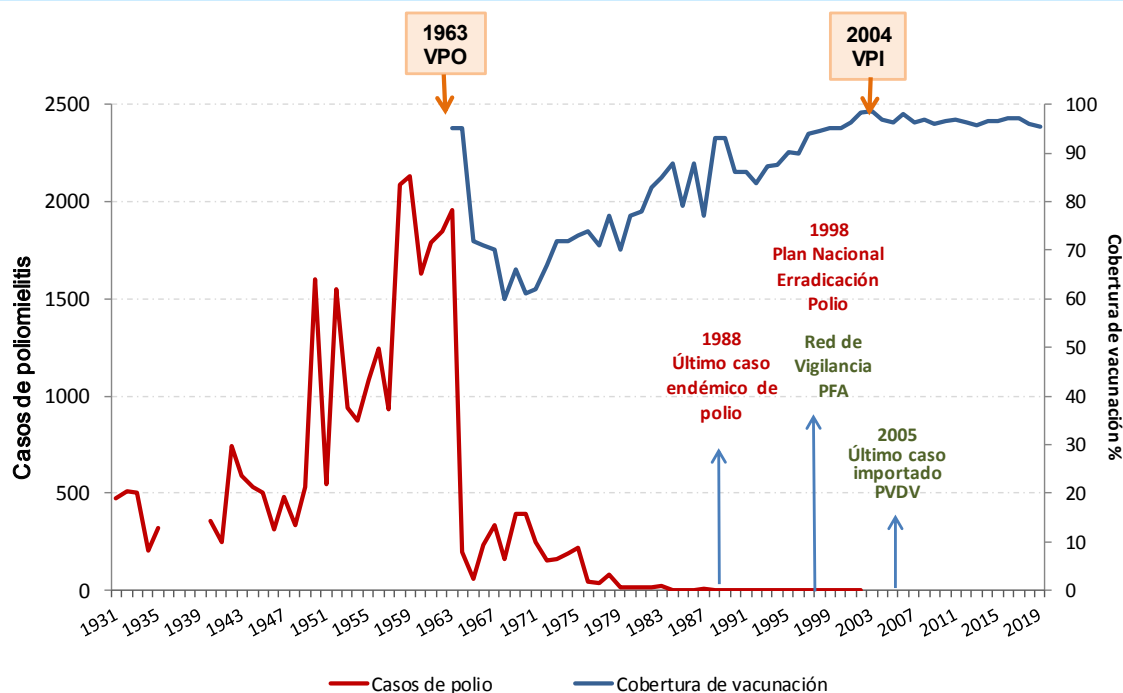
Figura 1. Casos de poliomiélitis y coberturas de vacunación. España, 1931-2019
